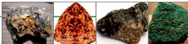
Uraninite
