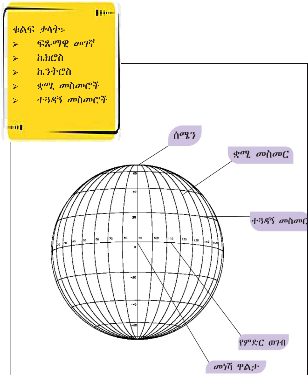
ሥዕል 2 በሉል ላይ ያሉ የሀሳብ መስመሮች ስያሜ
